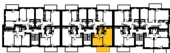
RZUT II PIĘTRA
